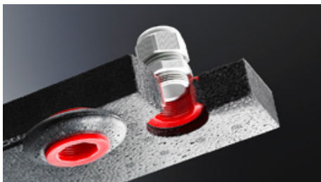
Partikelschaum-Verbundspritzgießen: Ein Verbundteil aus geschäumter und gespritzter Kunststoffkomponente kann in einem weiteren Schritt als Normteil integriert werden. Fotos: ARBURG
